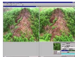
クラック図作成
