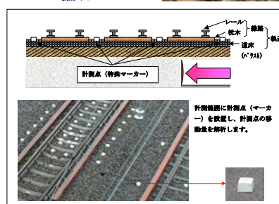
計測点 (特殊マーカー) の配置
